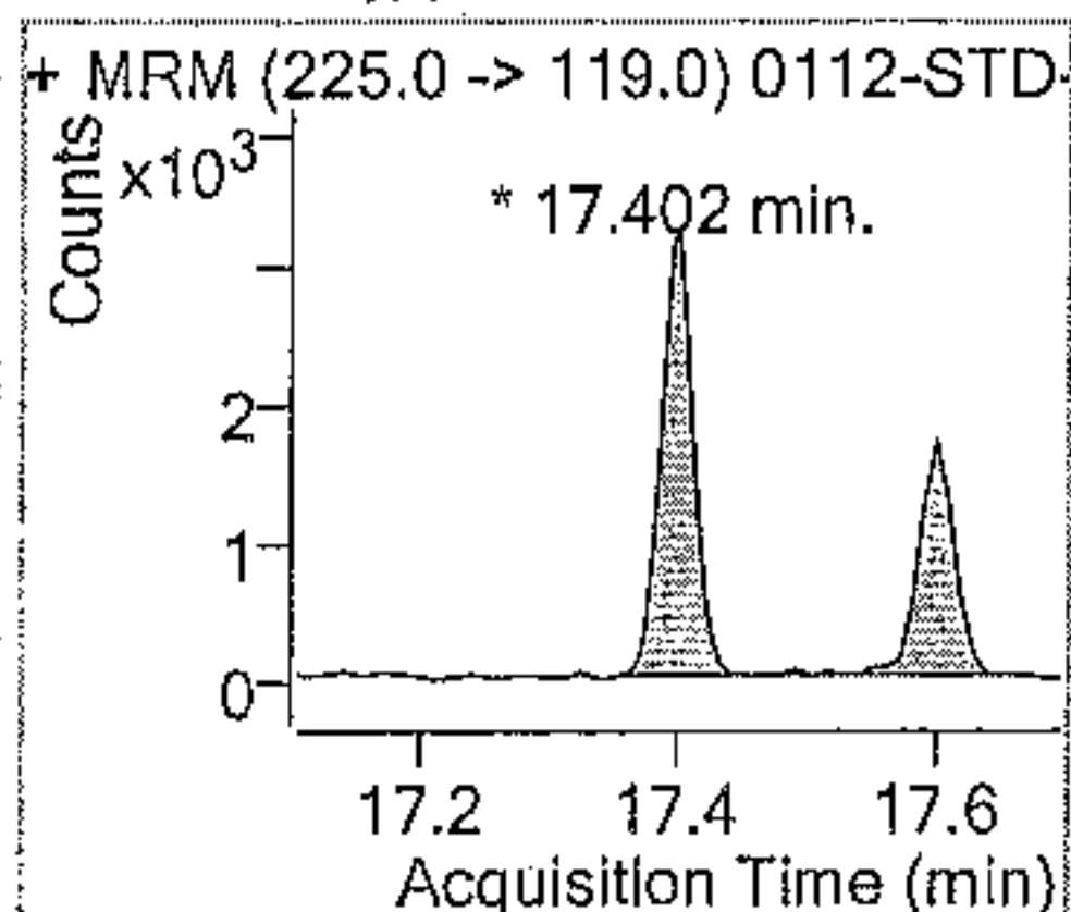
\lambda -Cyhalothrin 賽
