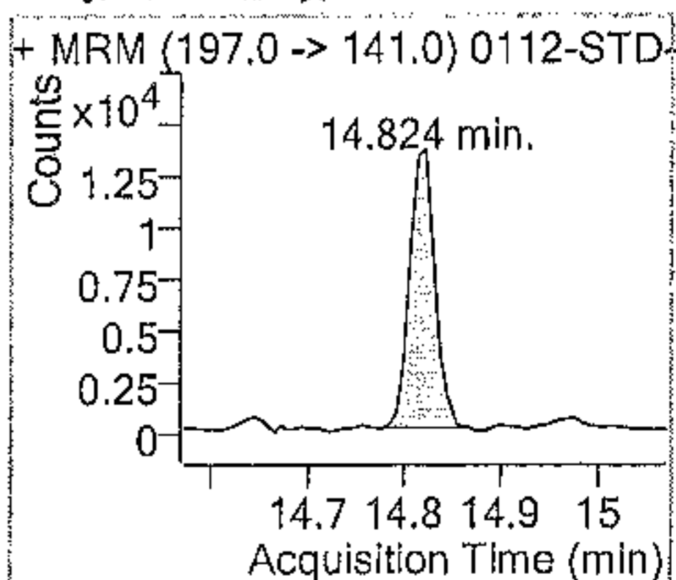
\lambda -Cyhalothrin 賽
