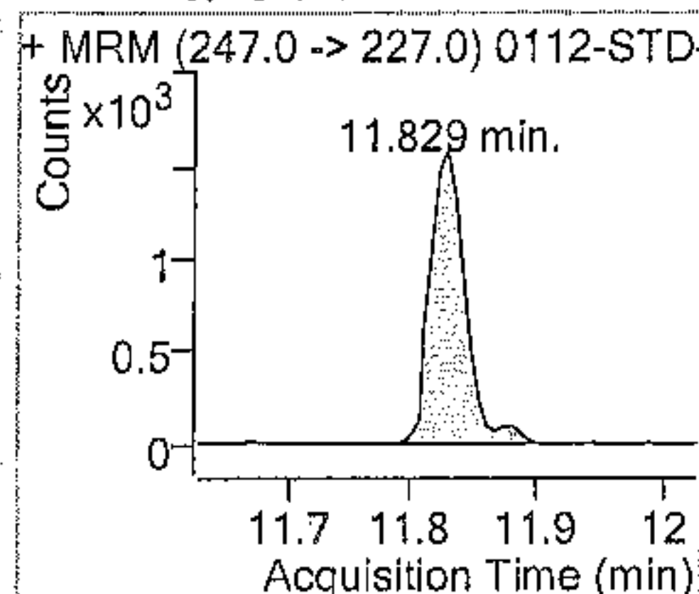
Fenvalerate 芬化
